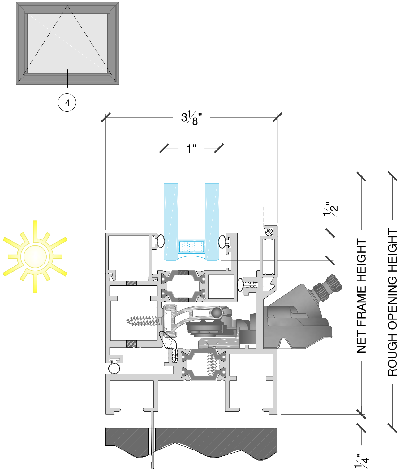
4 Awning Sill
